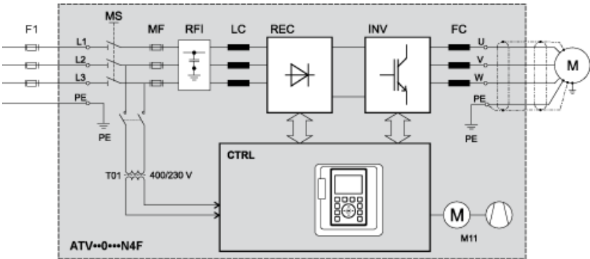
落地式驱动器电路图
