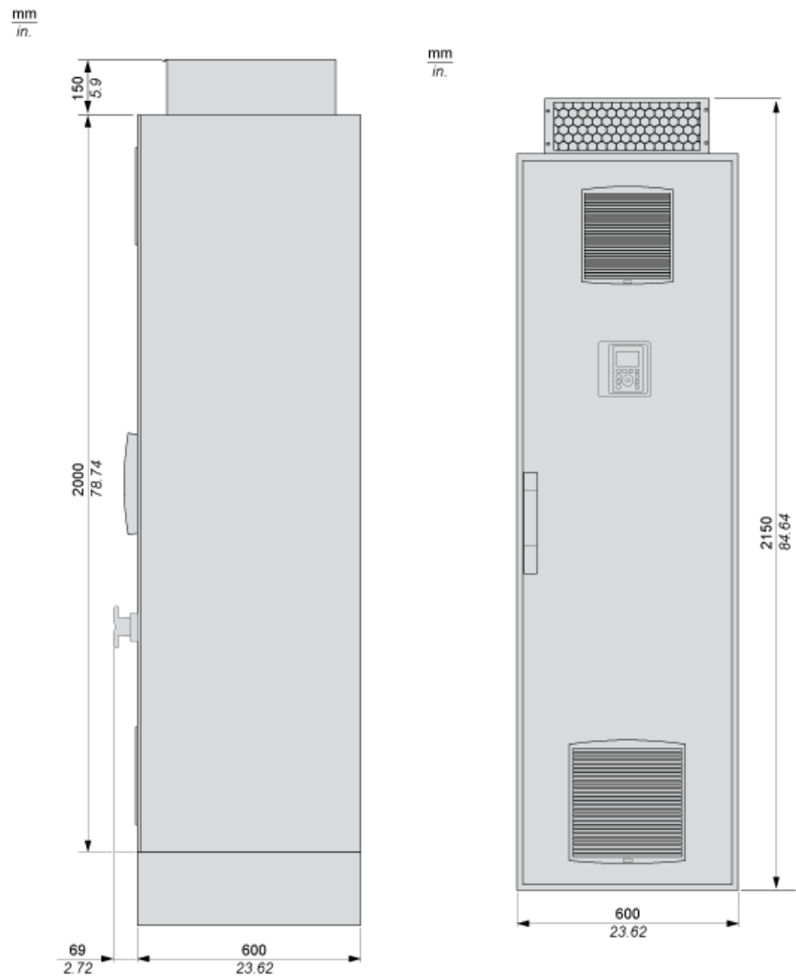
右侧视图和正面视图
