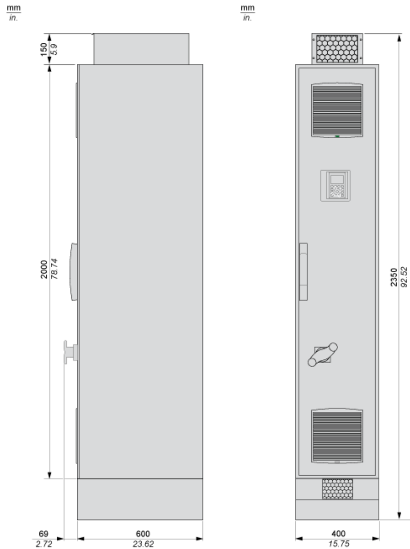
右侧视图和正面视图
