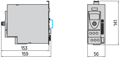
ABL 8BBU24200 和 ABL 8BBU24400 电池控制模块
