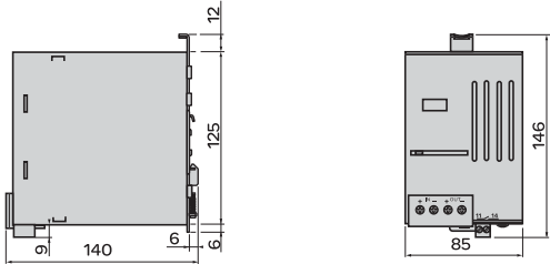
ABL 8BBU24200 电池控制模块
