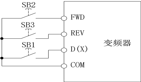
4. 三线制运转控制3示意图
