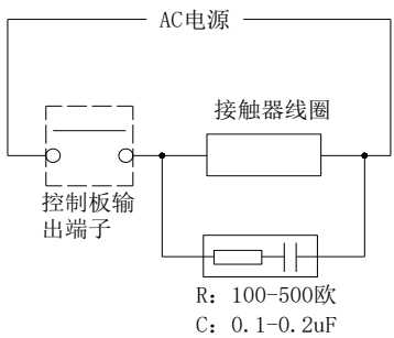
RC阻容吸收电路
