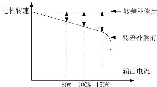
转差频率补偿示意图
