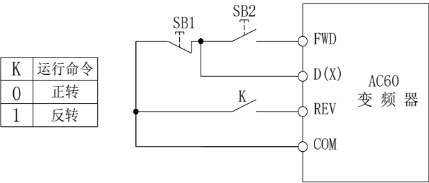
2. 三线制运转控制1示意图
