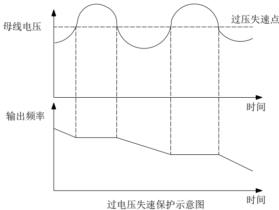
过电压失速保护示意图
