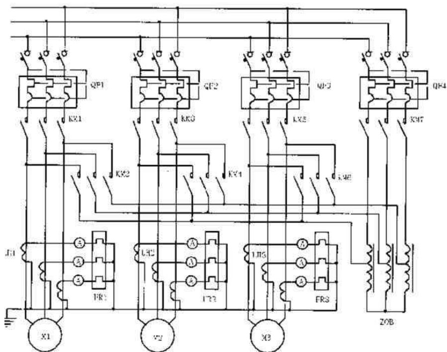
图 1 主电路图
