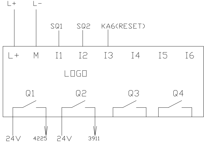
图 4 LOGO!接线图
